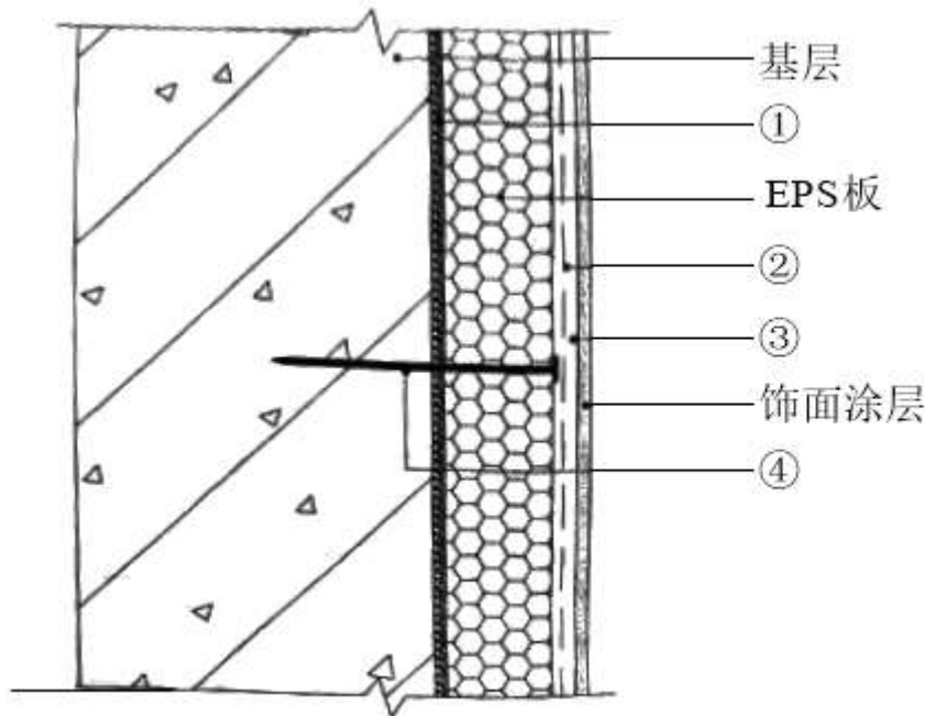
图 1-2 EPS 板薄抹灰构造图
